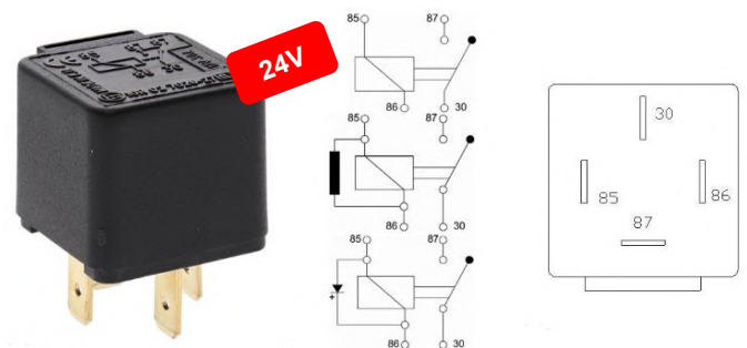
E020046 Relais 24V 20A 4 bornes
