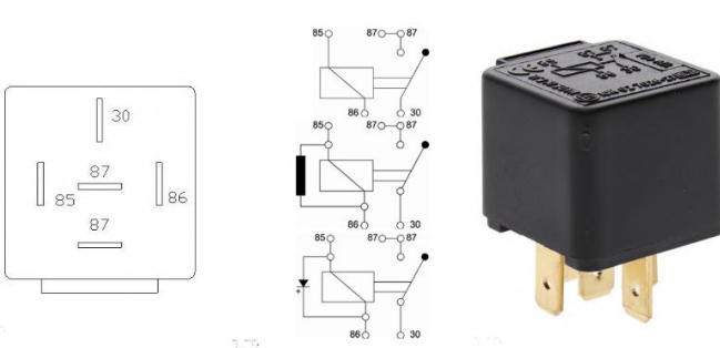
E020047 Relais 12V 40A 5 bornes
