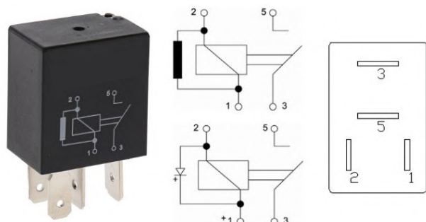
E020042 Micro-relais 12V 30A +résistance
