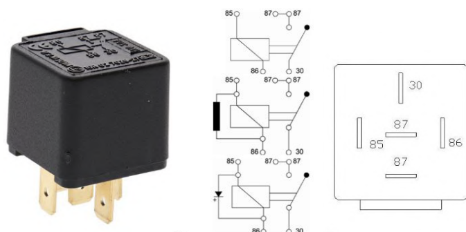
E020044 Mini-relais 5B 12V 30A Conditionnement sous blister
