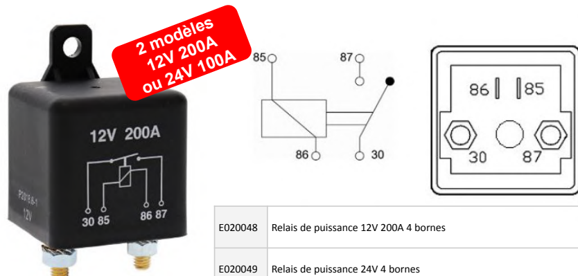
E020049 Relais de puissance 24V 4 bornes
