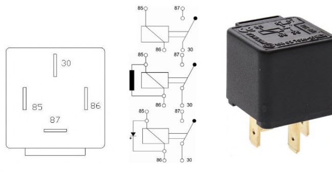
E020045 Mini-relais inverseur 4B 12V 30A Conditionnement sous blister
